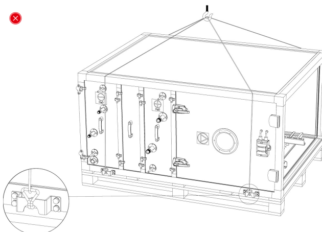
Pav. 9.2.2.2. Netaisyklingas VĮ sekcijos kėlimas naudojant kilpas (be medinių tarpiklių).
