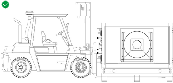
Pav. 9.2.3.1. Taisyklingas VJ sekcijos su atraminio padu kėlimas naudojant šakinį keltuvą.
