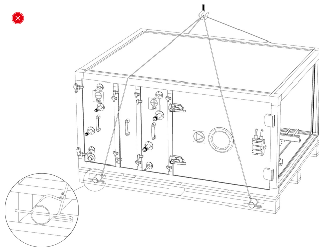
Pav. 9.2.1.4. Netaisyklingas VĮ sekcijos be atraminio pado kėlimas naudojant sijas (nėra medinių tarpiklių).
