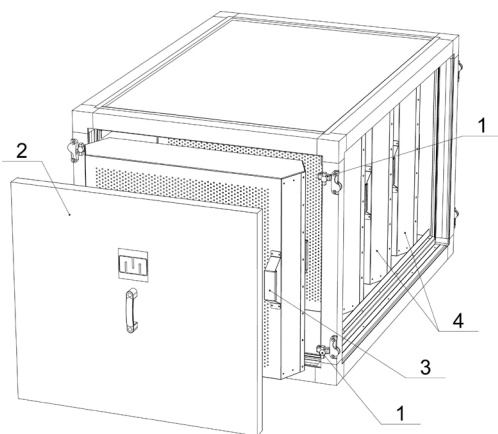
Pav. 8.2.1. Garso slopintuvo sekcija.
