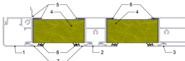
Pav. 5.2.1. AmberAir MD50 skerspjūvis.
