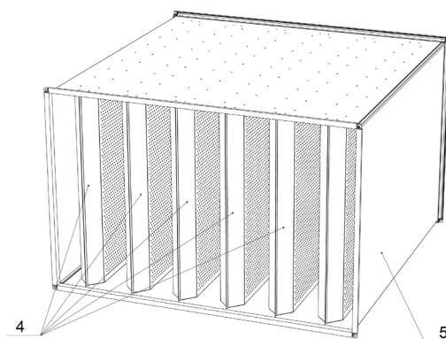
Pav. 8.2.2. Ortakinis garso slopintuvą
