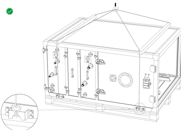
Pav. 9.2.2.1. Taisyklingas VĮ sekcijos kėlimas naudojant kilpas.
