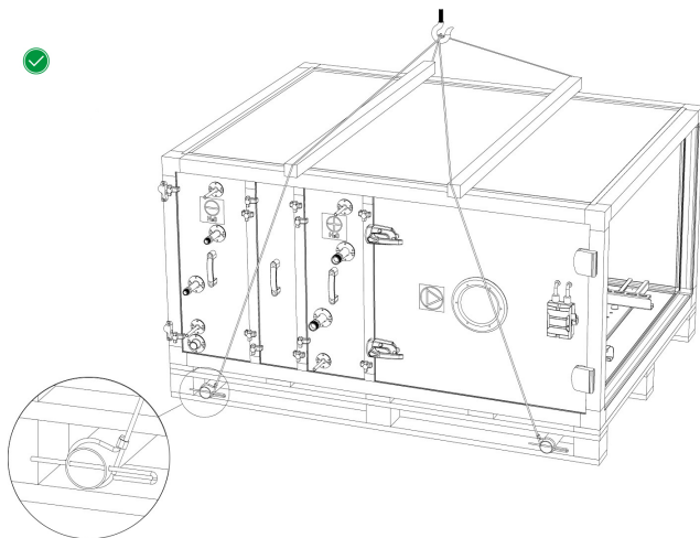
Pav. 9.2.1.3. Taisyklingas VĮ sekcijos be atraminio pado kėlimas naudojant sijas.
