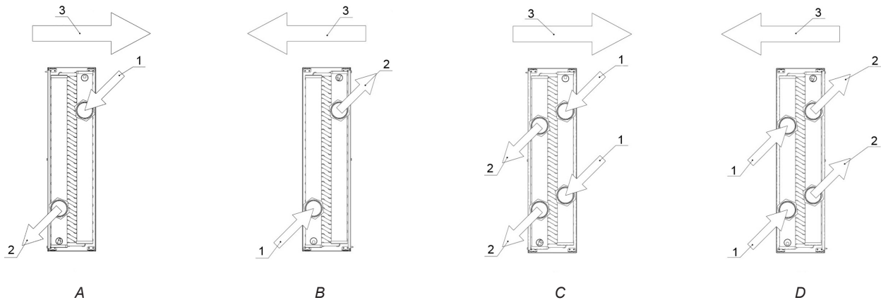
Pav. 6.3.1.2. (A, B) – Šildytuvo priešsrovinis pajungimas (vienas skysčio įleidimo ir išleidimo vamzdis).
