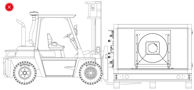
Pav. 9.2.3.2. Netaisyklingas VJ sekcijos su atraminio padu kėlimas naudojant šakinį keltuvą (sekcija nepilnai guli ant šakių).
