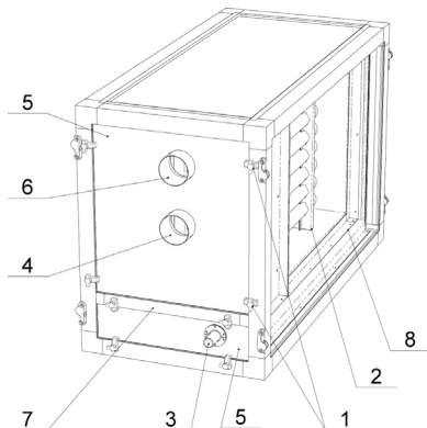
Pav. 6.3.6.1. Dujinio šildytuvo sekcija, montuojama patalpoje.
