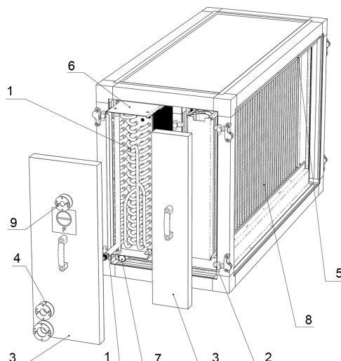
Pav. 6.3.3.5. Aušintuvo su išgaruojančiu šaltnešiu sekcija.
