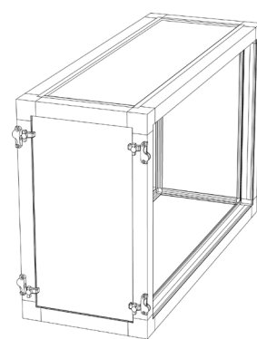
Pav. 6.8.3. D tipo aptarnavimo sekcija.
