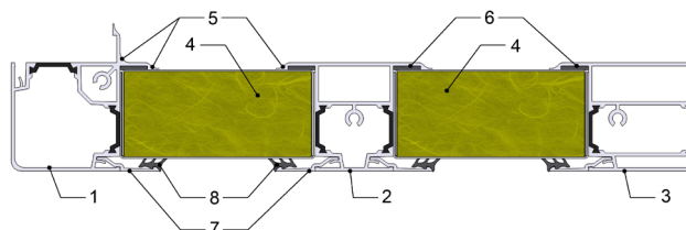
Pav. 5.2.2. AmberAir MD50+ skerspjūvis.
