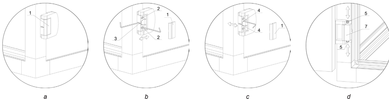
Pav. 9.5.3. (a, b, c, d) – AmberAir vyro suderinimas.
